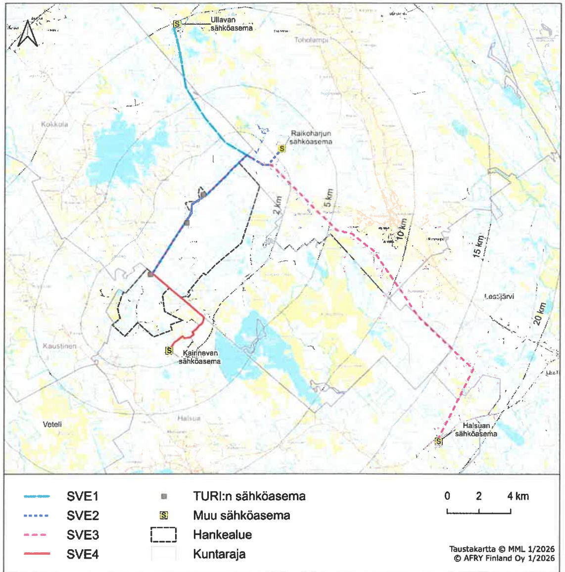
Kuva 1. Tuulivoimaloiden hankealue, sähköasemat ja sähkönsiirtoreitit vaihtoehdoissa SVE1-SVE4.
